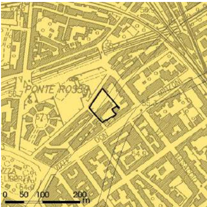
PERICOLOSITÀ SISMICA 1 2 3 4 3* 3**
