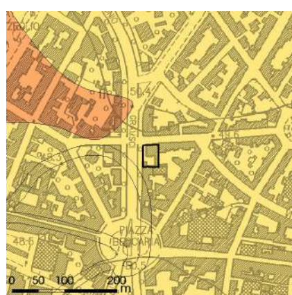
PERICOLOSITÀ SISMICA
